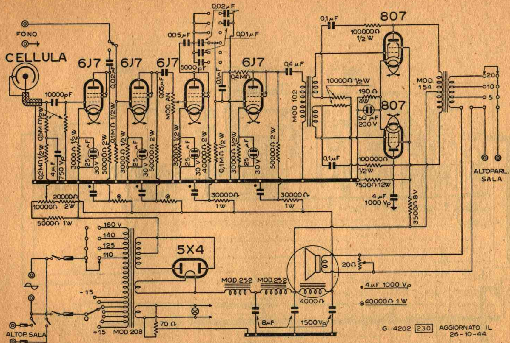
Lo schema elettrico dell'amplificatore Prevost mod. "302 ..."
